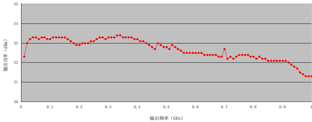
频谱特性图
